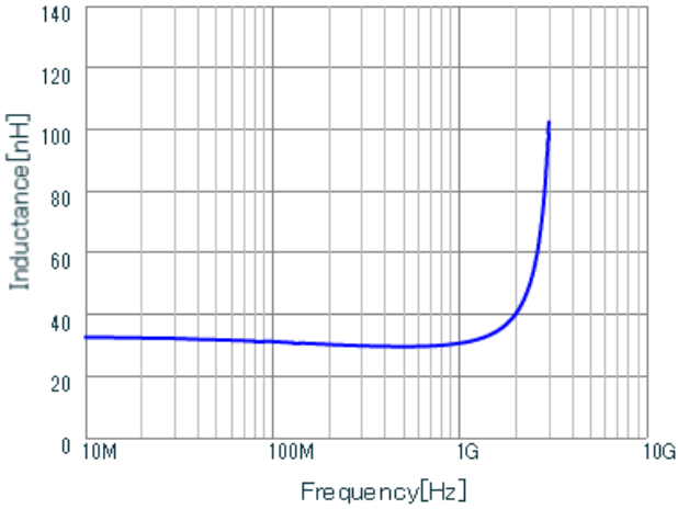
LQP02HQ33NH02 L.
