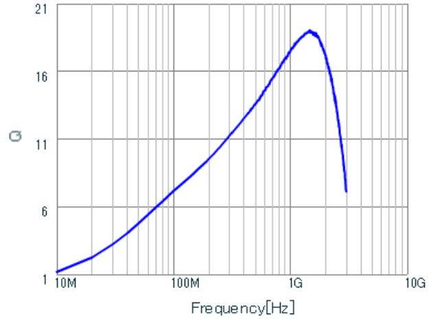
LQP02HQ33NH02 Q.
